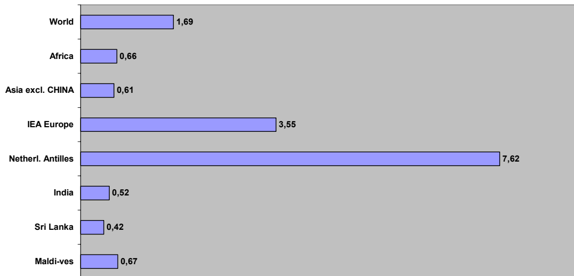
TPES/Capita
